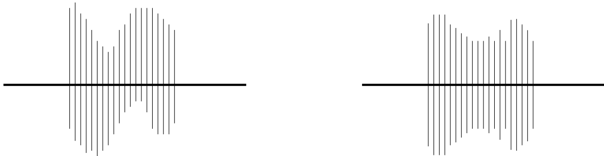
FIGURE 3. Représentation schématique de la symétrisation de Steiner
