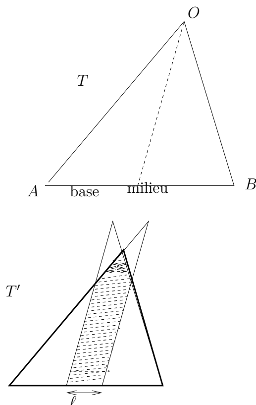
FIGURE 9. Réduction de l'aire sans perte de directions
