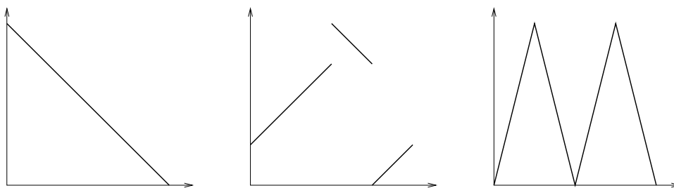
FIGURE 3. Quelques graphes de transformations préservant la mesure de Lebesgue
